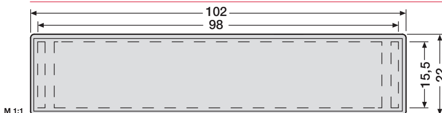
Sichtglas mit 2 Haltekeilen – Einbau ab 1970 –
