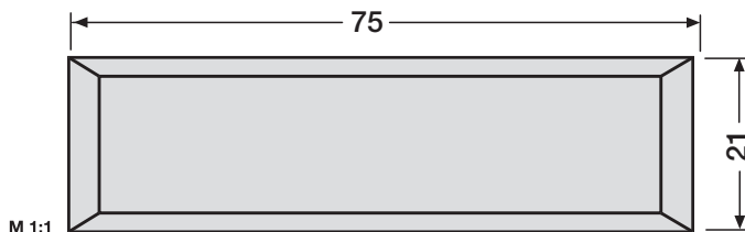
Namensschild -Auslaufmodell- SEKO 75 x 21 Verkauf solange Vorrat reicht von vorne auswechselbar für Ausstanzung 71,3 x 19,3 mm, alternatives preisgünstigeres Ersatzprodukt (andere Optik): Namensschild 92 (siehe Seite 25) Best.-Nr. 97-9-82016
