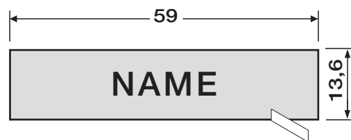
RSA2-kompakt Namensschild einlage aus grauem Kunststoff gravierbar, für 97-9-85339, 97-9-85321 u. RSA2-kompakt-Block Seite 11 ohne Gravur 97-9-87245 dito mit Gravur, Schriftfarbe weiß 90-3-00023
