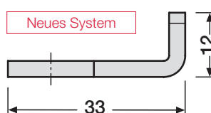
Riegel gekröpft – Auslaufmodell – für 3-Punkt-Verriegelung Serienkästen
