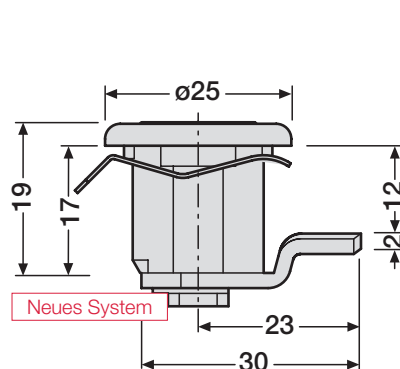
Zylinderschloss RE Schließung 1-200, inkl. 2 Schlüssel, Einbau ab 1990 Passender Ersatz:
