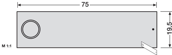
ALU-RSA2-kompakt Namensschild ohne Gravur, 97-9-85338 für 97-9-85319 und RSA2-kompakt-Block Seite 10 dito Edelstahl Ausführung ohne Gravur, für 97-9-85317 97-9-85337 und RSA2-kompakt-Block Seite 10
