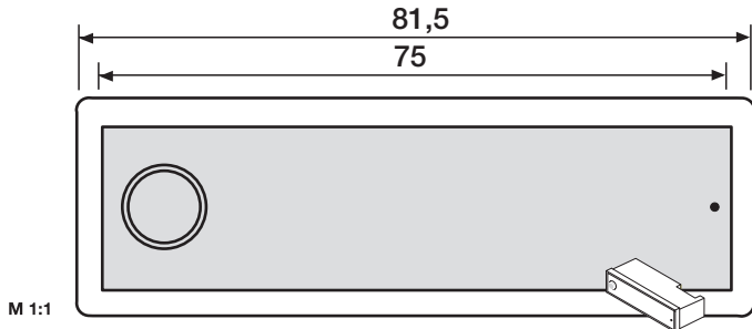
ALU-RSA2-kompakt Klingeltaster 97-9-85319 – Einbau ab 2009 – ohne Gravur, mit Montagegehäuse, Anschluss 12 – 24 V, inkl. LED-Beleuchtungsring 0,12 Watt AC/DC 12 V dito Edelstahl Ausführung 97-9-85317 Passende RSA2-Beleuchtungen siehe Seite 27.
