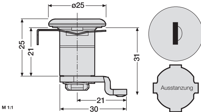
Zylinderschloss ER – Einbau ab 2006 – Schließung 1-100 inkl. 2 Schlüssel, für Modellgruppe 22
