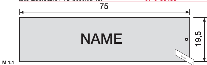
ALU-RSA2 Namensschild mit schwarzer Gravur
