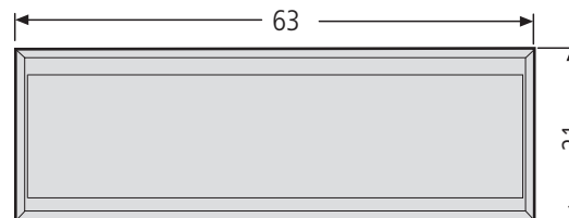
Namensschild – Nicht mehr lieferbar – 63 x 21 mm, glasklar, Ausstanzung 60 x 18 mm
