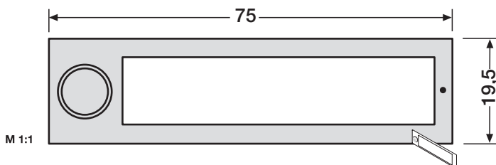
Kunststoff-RSA2-kompakt Namensschildabdeckung 97-9-85339 ohne Gravur für 97-9-85321 und RSA2-kompakt-Block Seite 11 Einlage max. 59 x 13,6 x 1 mm
