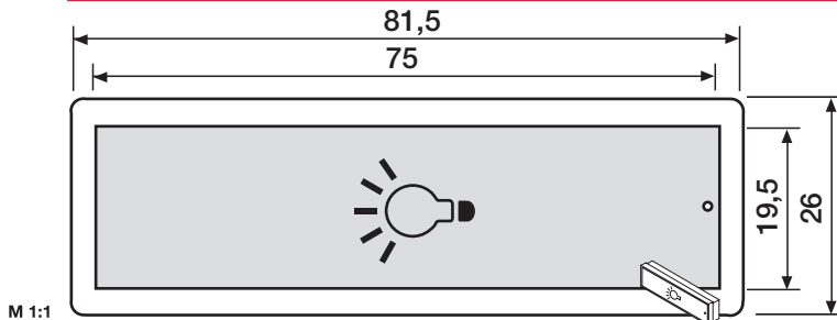
ALU-RSA2 Lichtschild mit Gravur
