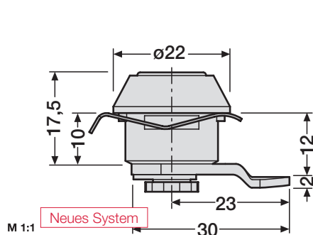
Zylinderschloss FH Schließung 1-200, inkl. 2 Schlüssel Passender Ersatz:
