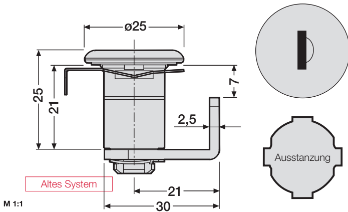
Zylinderschloss ER – Einbau ab 2006 – Schließung 1-50 inkl. 2 Schlüssel
