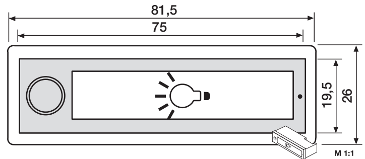
Kunststoff-RSA2-kompakt Lichttaster 97-9-85322 – Einbau ab 2009 – Einlage mit Symbol Glühbirne, mit Montagegehäuse, Anschluss 12 – 24 V, inkl. LED-Beleuchtungsring 0,12 Watt AC/DC 12 V
