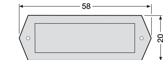
Namensschild ALU-Rahmen EV1 Verkauf solange Vorrat reicht 58 x 20 mm
