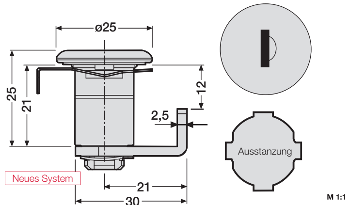
Zylinderschloss ER – Einbau ab 2006 – Schließung 1-400 inkl. 2 Schlüssel, 1 Satz (50 Stück)
