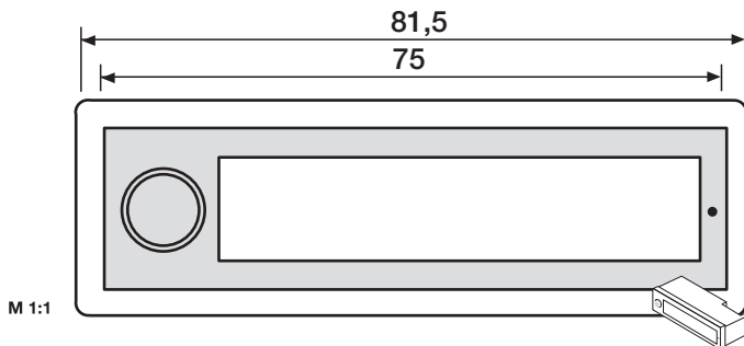
Kunststoff-RSA2-kompakt Klingeltaster 97-9-85321 – Einbau ab 2009 – mit Montagegehäuse, Einlage max. 59 x 13,6 x 1 mm, Anschluss 12 – 24 V, inkl. LED-Beleuchtungsring 0,12 Watt AC/DC 12 V
