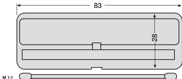
Klappenhalter Verkauf solange Vorrat reicht mit Torsionsfeder, 83 x 28 mm
