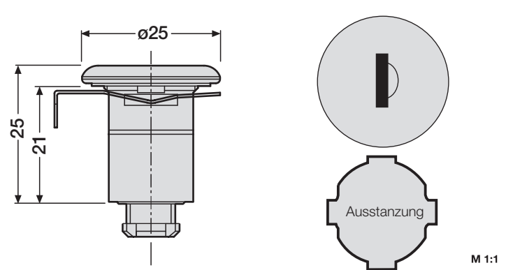
Zylinderschloss ER – Einbau ab 2006 – Schließung 401-500 inkl. 2 Schlüssel, ohne Riegel
