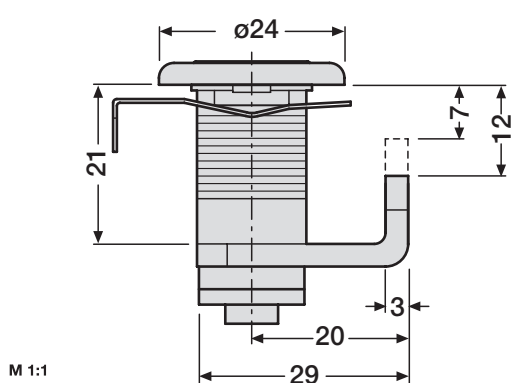
Zylinderschloss 448 – Einbau seit 1993 – Schließung EL 1-200 inkl. 2 Schlüssel, mit zwei Riegel 1 Satz (50 Stück) Zylinderschloss 448 Schließung EL 500 inkl. 2 Schlüssel, mit zwei Riegel, Einbau in Installationskästen, Ersatz für TX01, RX01, 2H 500-Schlösser
