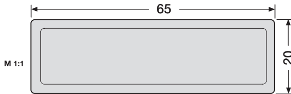
Namensschild Verkauf – Nicht mehr lieferbar – Größe 65 x 20 mm, Ausstanzung 60,8 x 17,8 mm
