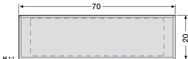
Namensschild Verkauf solange Vorrat reicht 70 x 20 mm, Ausstanzung 67 x 17 mm
