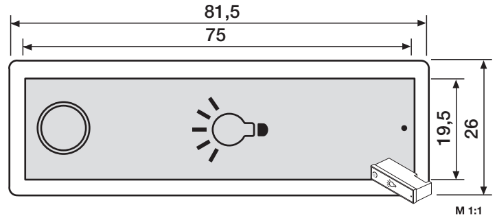
ALU-RSA2-kompakt Lichttaster mit Gravur 97-9-85320 – Einbau ab 2009 – Symbolgravur Glühbirne, mit Montagegehäuse, Anschluss 12 – 24 V, inkl. LED-Beleuchtungsring 0,12 Watt AC/DC 12 V dito ALU mit grauer Laserbeschriftung 97-9-92506 dito Edelstahl Ausführung mit Gravur 97-9-85318 Laserbeschriftung 97-9-92505 Passende RSA2-Beleuchtungen siehe Seite 27.
