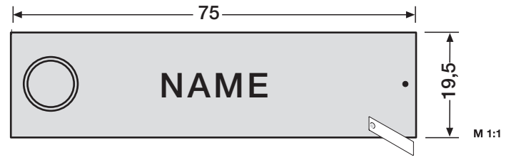
ALU-RSA2-kompakt Namensschild 90-3-00026 mit schwarzer Gravur*, für 97-9-85319 und RSA2-kompakt-Block Seite 10 dito ALU mit grauer Laserbeschriftung* 90-3-00045 dito Edelstahl Ausführung mit Gravur* 90-3-00025 mit weißer Gravur*, für 97-9-85317 u. RSA2-kompakt-Block Seite 10 dito Edelstahl Ausführung mit grauer Laserbeschriftung* 90-3-00044
