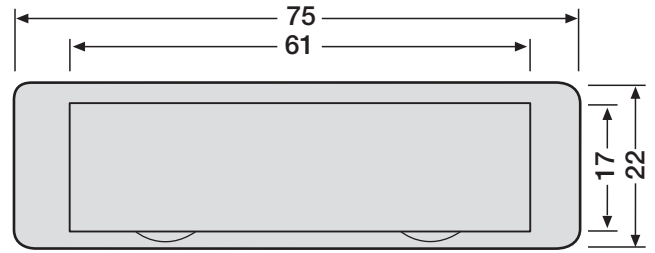
Namensschild 92 – Einbau bis 2009 –
