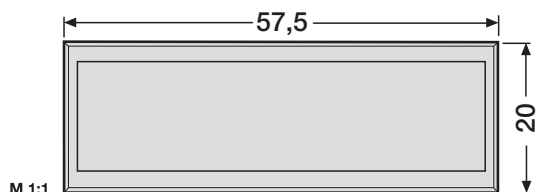
Namensschild Verkauf solange Vorrat reicht grau, 57,5 x 20 mm
